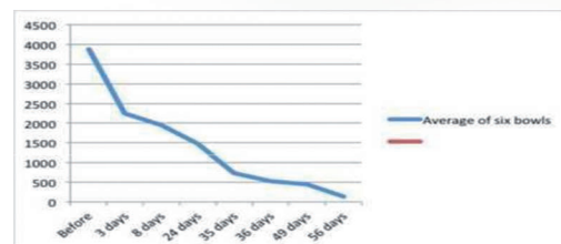
Effet sur la croissance des bactéries dans un lave-vaisselle
